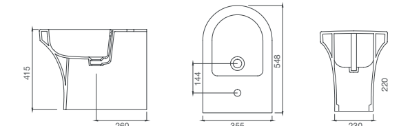
SO02BDE00 SOLE DUVARA ASMA BIDE
