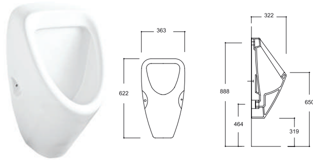
TP04PSR00 | TP04PSR00 FOTOŞEL UYUMLU PİSUVAR | URINAL
