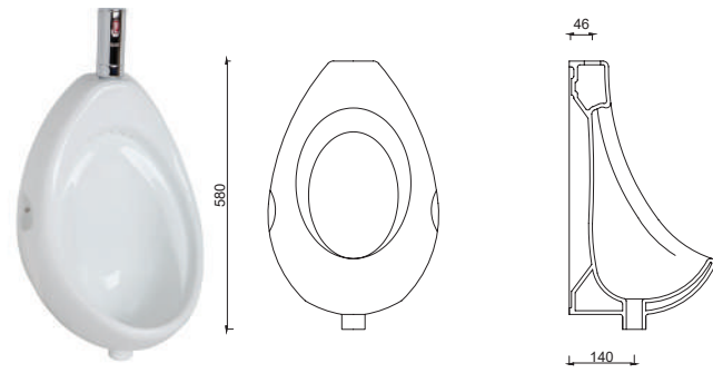
TP07PSR00 | TP07PSR00 FOTOŞEL UYUMLU PİSUVAR | URINAL
